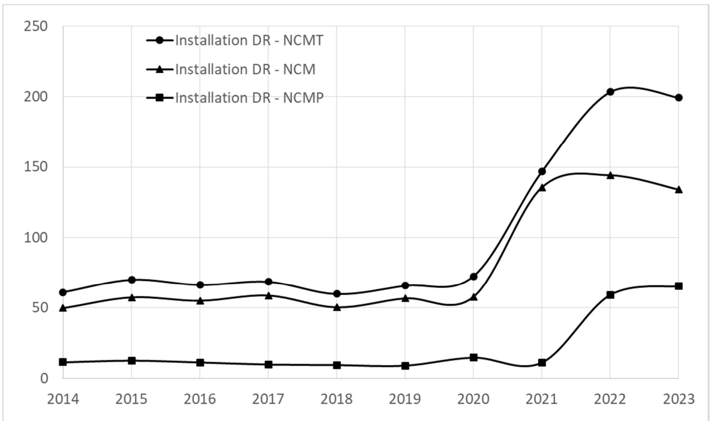
Figure 18 : Evolution du nombre de NCM, NCMP et NCMT constatées pour 100 contrôles d'installations de mammographie numérique de type DR
